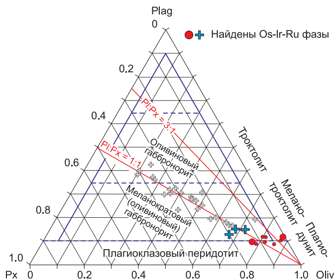
Рис. 2. Вариации состава оливковых габброноритов и плагноклазовых перидотитов подошвы Йоко-Довыренского массива.
