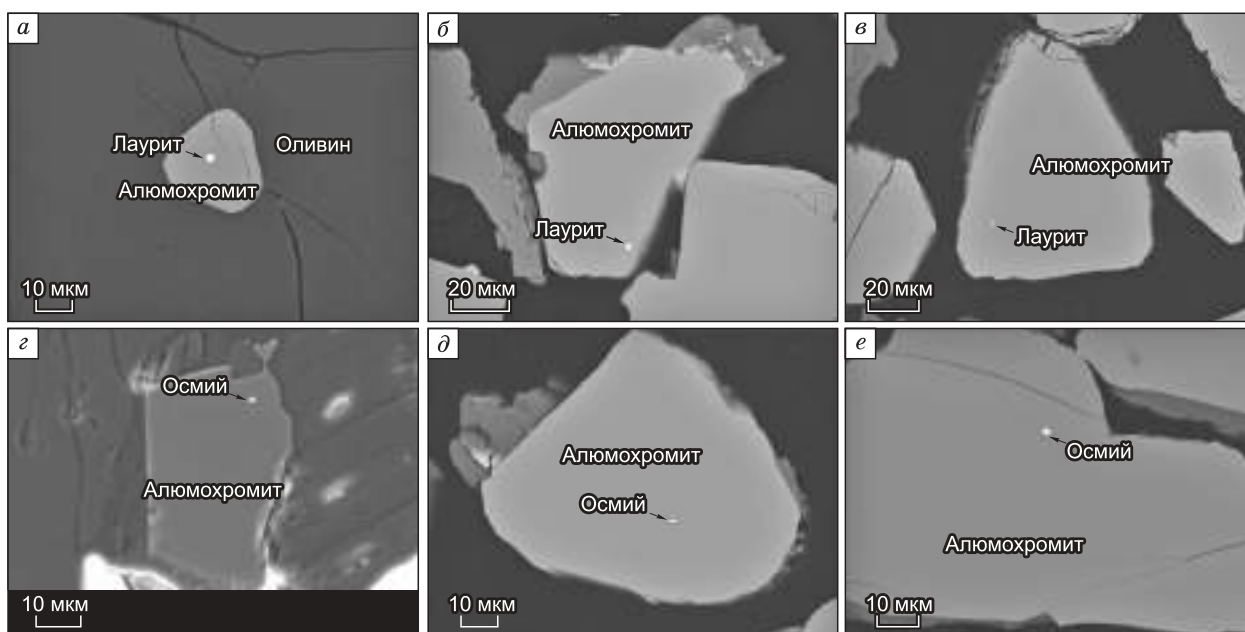
Рис. 6. Включения Os-Ir-Ru фаз в алюмохромите из плагиоферидотитов Йоко-Довыренского массива:
