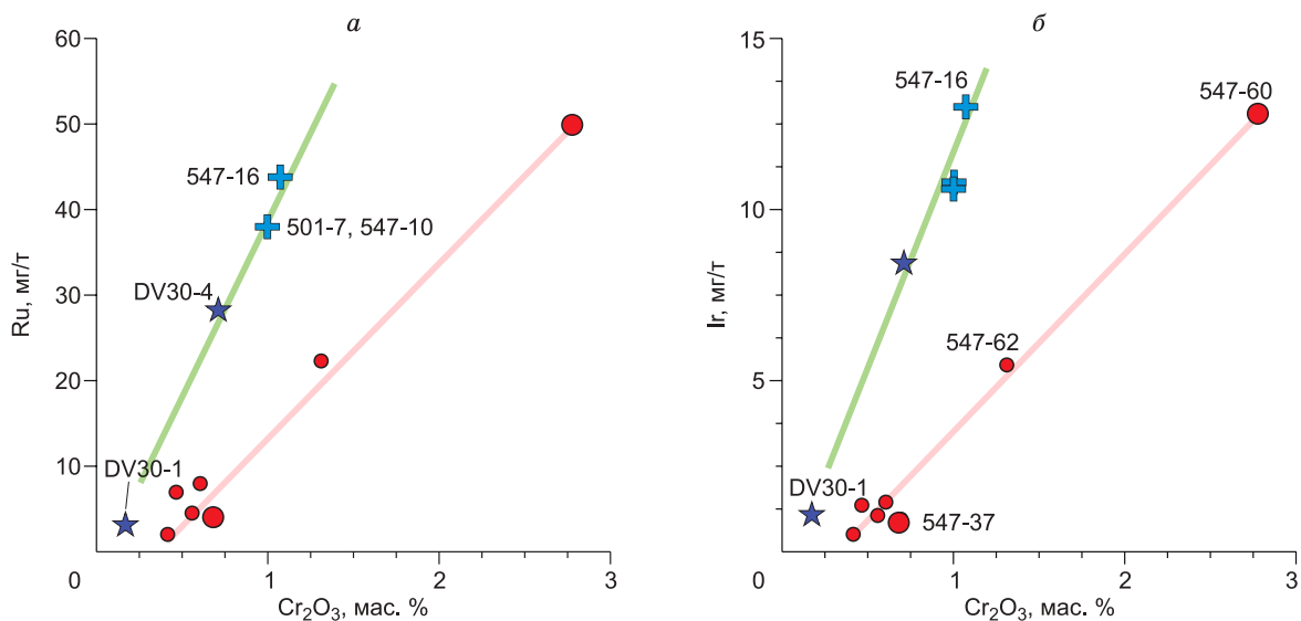
Рис. 7. Зависимость валовых содержаний Ru и Ir от \text{Cr}_2\text{O}_3 для изученных плагиоперидотитов.
