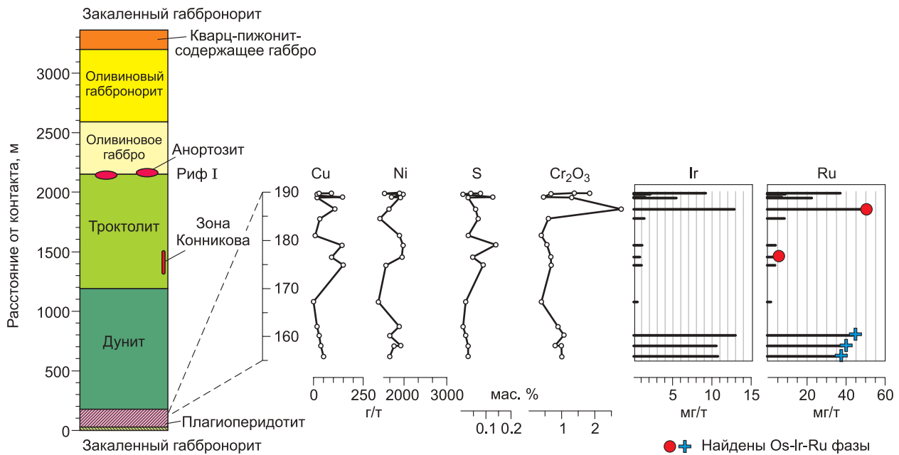
Рис. 1. Строение Йоко-Довыренского массива [Ariskin et al., 2016] и распределение серы, \text{Cr}_2\text{O}_3 , Cu, Ni, Ir и Ru в зоне перехода от плагиперидотитов к плагноклазсодержащим дунитам.
